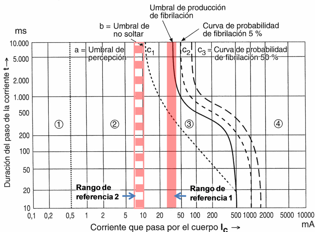
Figura 1. Zonas tiempo/corriente de los efectos de las corrientes alternas (de 15 Hz a 150 Hz) sobre los seres humanos.
