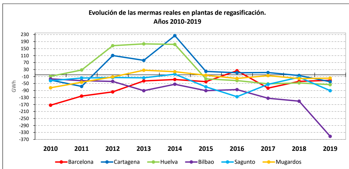
Figura 3: Evolución de las mermas reales en las plantas de regasificación del sistema gasista español (años 2010-2019).
