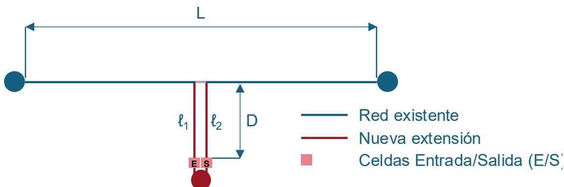
Figura 2. Incremento de longitud de línea existente en conexión en Entrada/Salida (E/S)
