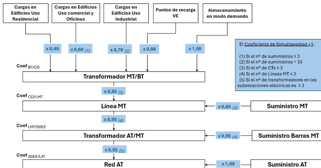
Figura 4. Esquema de aplicación de los coeficientes de simultaneidad
