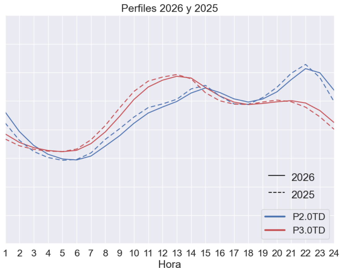
Gráfico 1. Comparativa del promedio de los perfiles P2.0TD y P3.0TD aplicables a 2026 y 2025.
