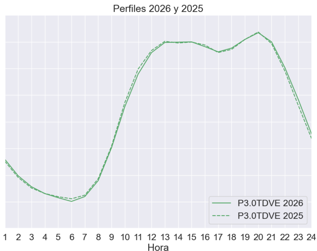
Gráfico 2. Comparativa del promedio de los perfiles P3.0TDVE aplicables a 2026 y 2025.
